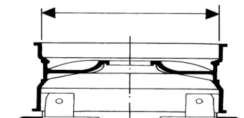
Ruote in lega Alloy rim wheels
